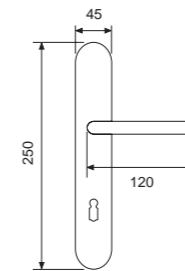
21022P - OLV Handle on plate Maner cu placa
