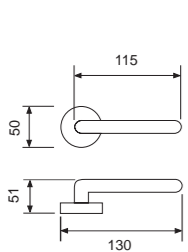
21024R04 - OLV Handle on rose Maner cu rozeta
