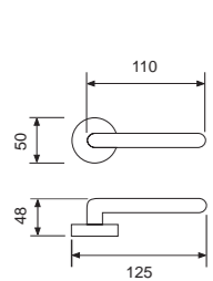
21077R04 - OLV Handle on rose Maner cu rozeta
