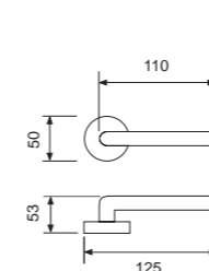
21034R04 - OGR Handle on rose Maner cu rozeta
