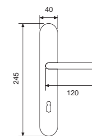
21020P - OLV Handle on plate Maner cu placa
