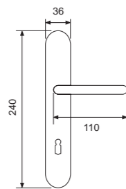
21192P - OLV Handle on plate Maner cu placa
